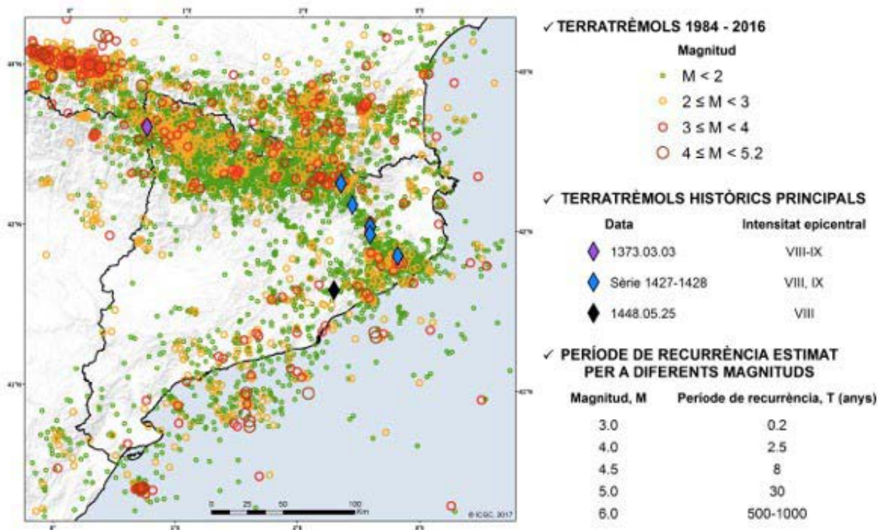
Figura 1.- Mapa de la sismicitat de Catalunya. Els períodes de recurrència ens indiquen que podem esperar, per exemple, uns 5 terratrèmols de magnitud 3 cada any o un de magnitud 4.5 cada 8 anys.
