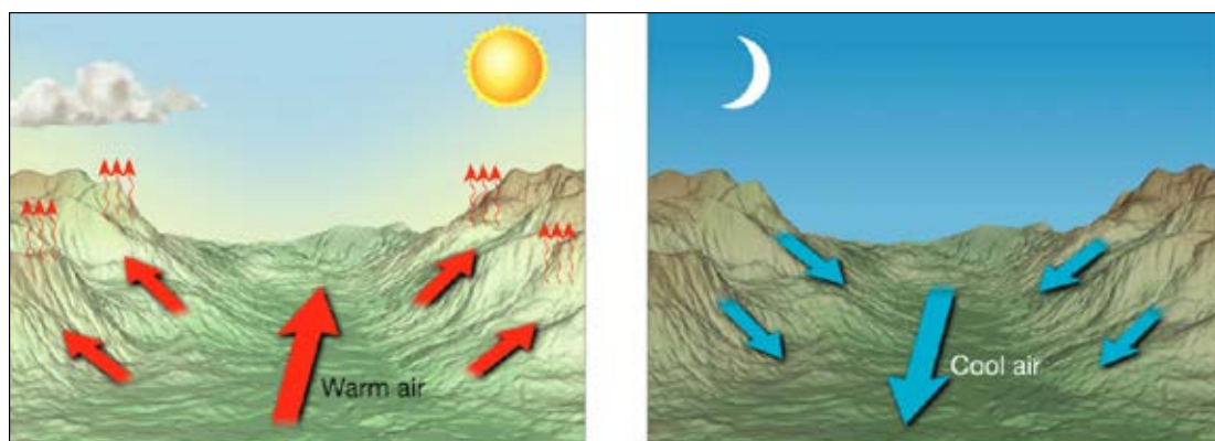
Figura 4: Circulacions locals que es produeixen a les muntanyes durant el dia i durant la nit.
